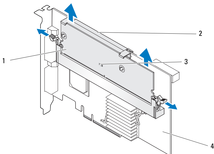
Figura 1. Ubicación del LED de caché con datos pendientes del adaptador PERC x/E
